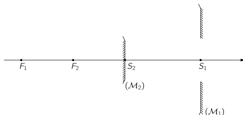
FIGURE 4 – Schéma de principe d'un télescope type Schmidt-Cassegrain.
