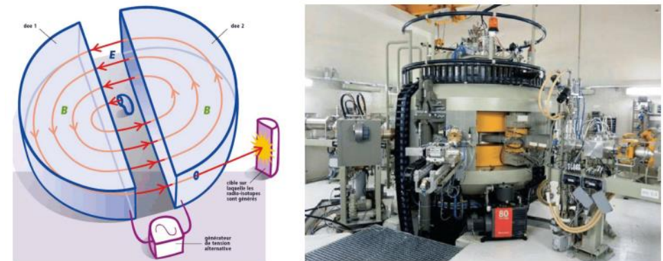
Figure 3 – Structure d'un cyclotron.
