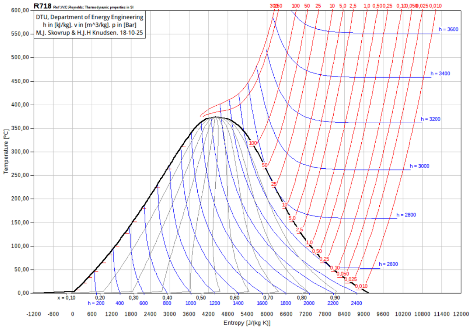
Figure 18 – Diagramme entropique de l'eau.
