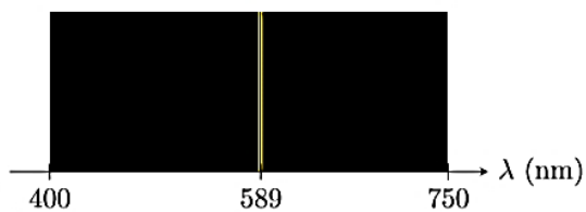
(a) Lampe à vapeur de sodium
