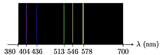
(b) Lampe à vapeur de mercure
