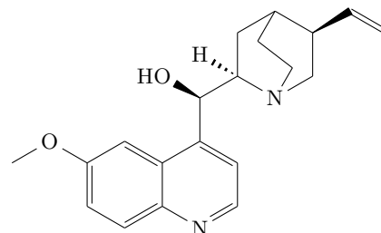
quinine (antipaludéen)
