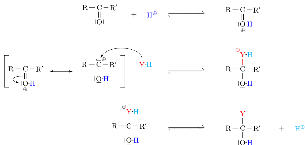
FIGURE 6 – Mécanisme d'une addition nucléophile A_H + A_N en milieu acide.
