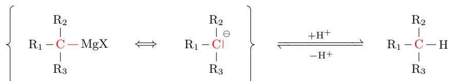
FIGURE 20 – Caractère de pseudo-carbanion fortement basique d'un organomagnésien.
