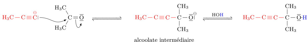
FIGURE 15 – Mécanisme de l'addition d'un ion alcynure sur le groupe carbonyle.
