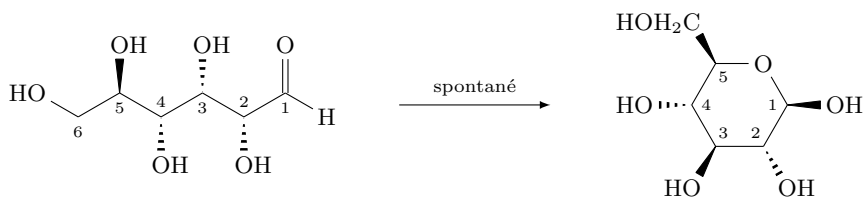
FIGURE 3 – Formation du glucopyranose par cyclisation du glucose.
