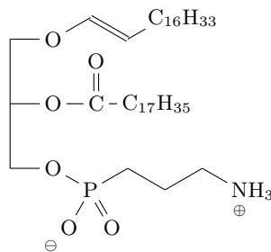
un plasmalogène
