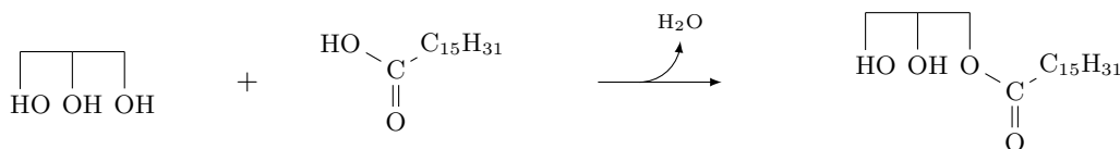
FIGURE 6 – Réaction d'estérification.
