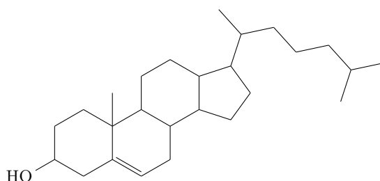
cholestérol
