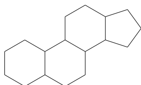
stérane
