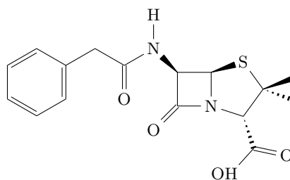
pénicilline G
