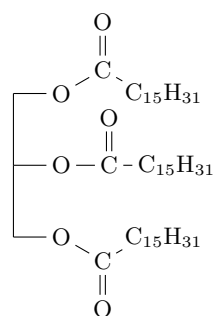
tripalmitylglycérol
