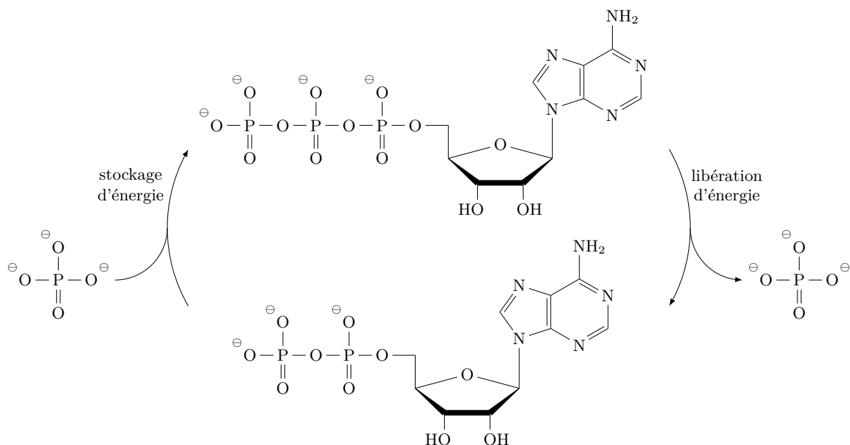
FIGURE 8 – Interconversion de l'ADP en ATP.
