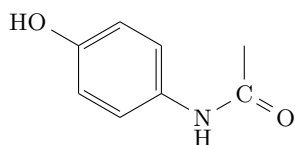
paracétamol (artificiel)
