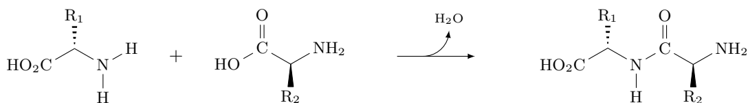
FIGURE 5 – Association de deux acides aminés par une liaison peptidique.
