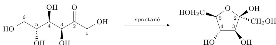
FIGURE 2 – Formation du fructofuranose par cyclisation du fructose.
