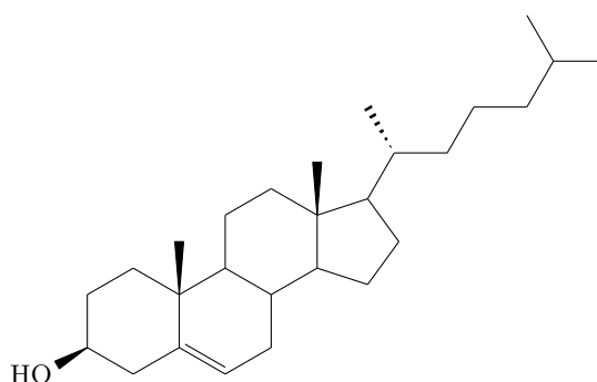
cholestérol
