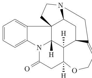
strychnine (naturelle)
