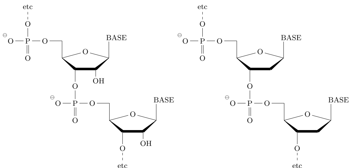
FIGURE 9 – Structure d'un brin d'ARN et d'un brin d'ADN.
