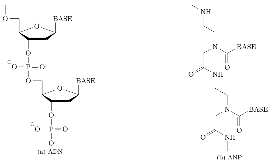
FIGURE 1 – L'ADN et son homologue synthétique l'ANP.
