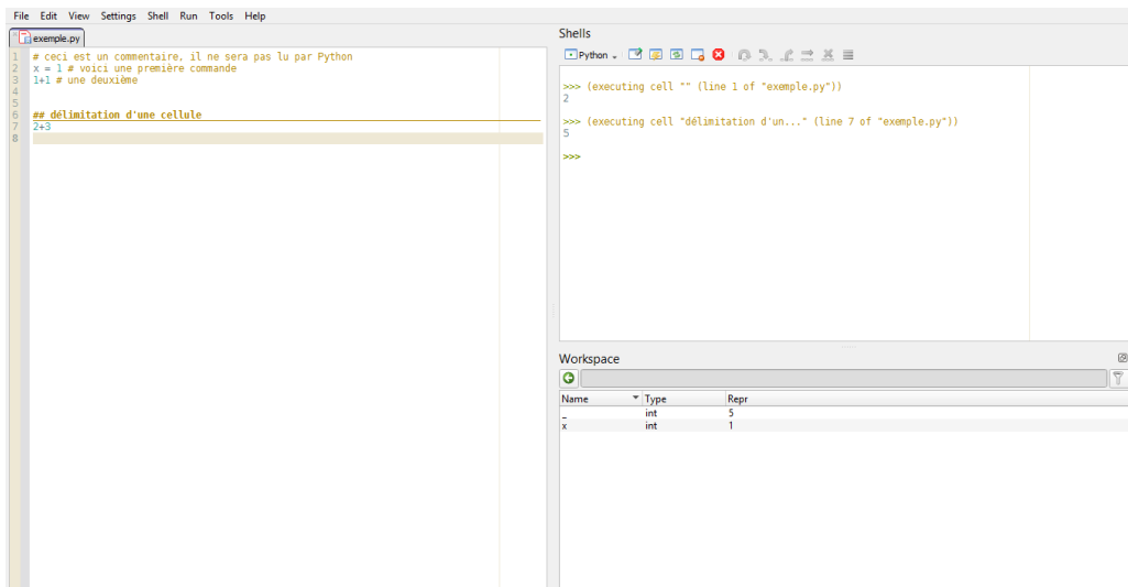
FIGURE 3 – L'IDE Pyzo
