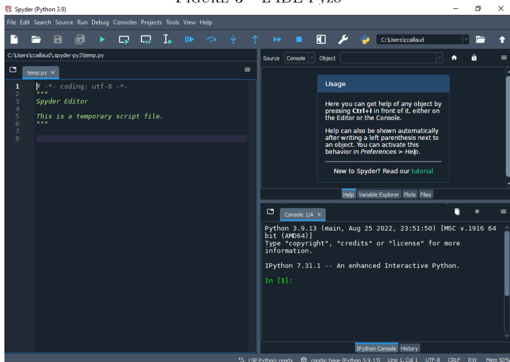
FIGURE 4 – L'IDE Spyder
