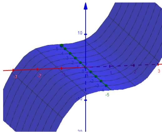
FIGURE 5 – Le point (0, 0) est point critique mais pas extremum local de f : (x, y) \longmapsto x^3
