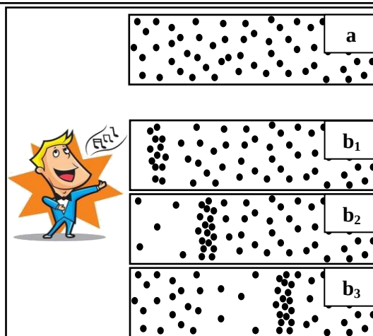
Doc 3 : Disposition moyenne des molécules présentes dans l'air : (a) en absence de son ; (b) quand un son bref est émis en b_1 puis se propage en b_2 et b_3 .
