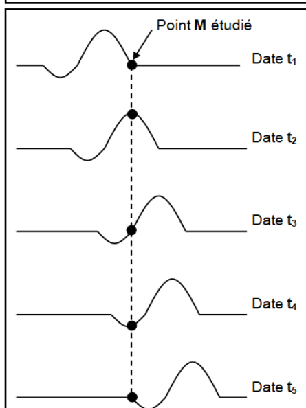
Doc 1 : Profil spatial d'une vague au cours du temps
