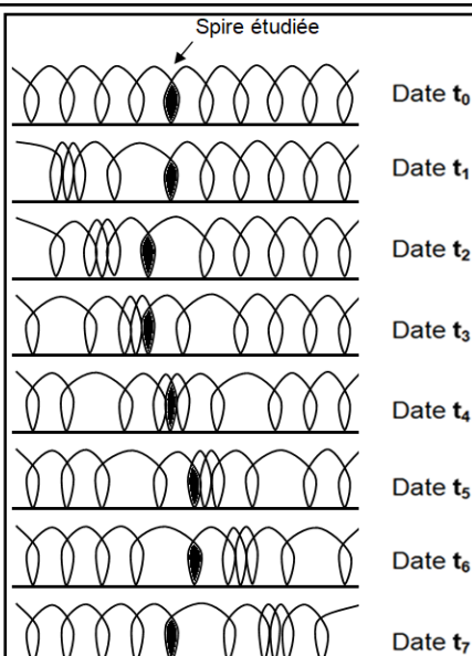
Doc 2 : Profil spatial d'un ressort au cours du temps
