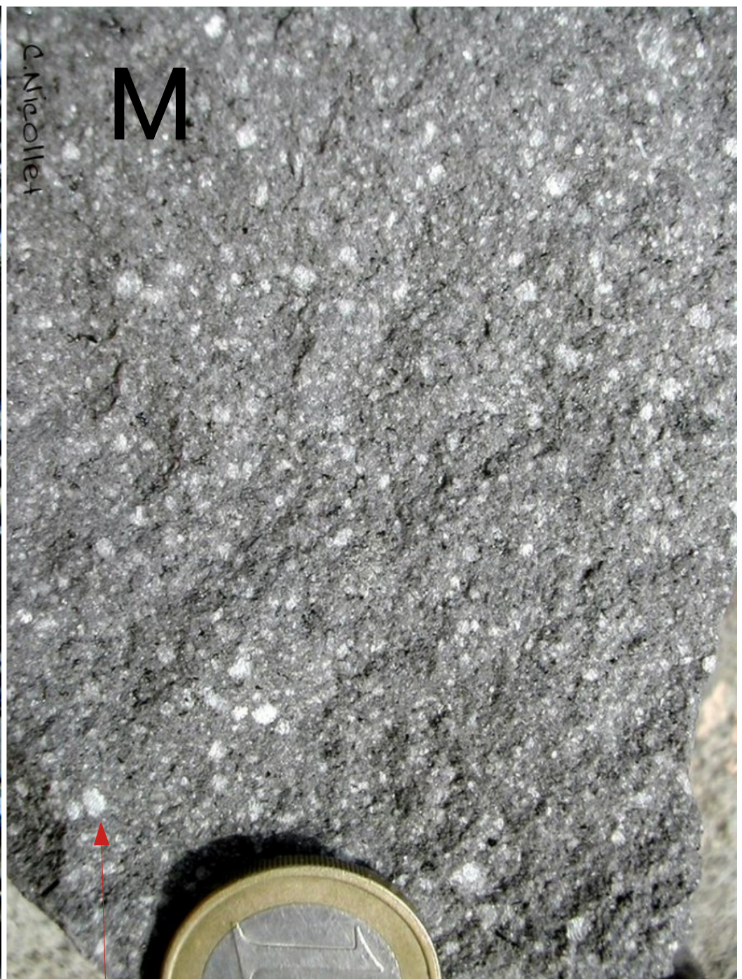
plagioclase
