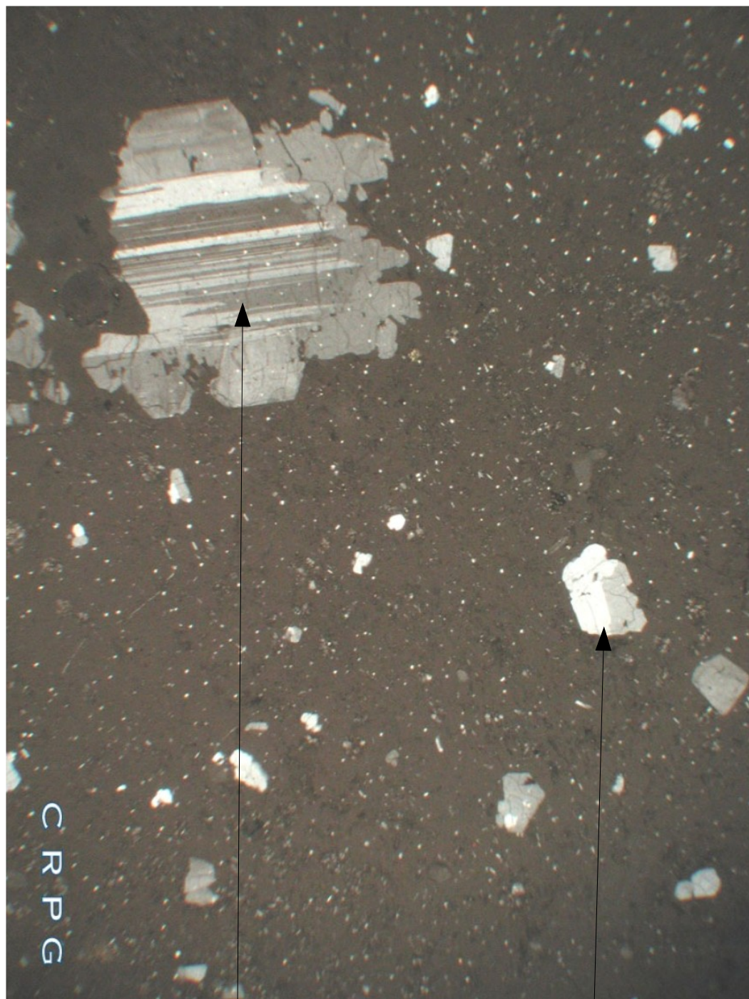
Plagioclase
