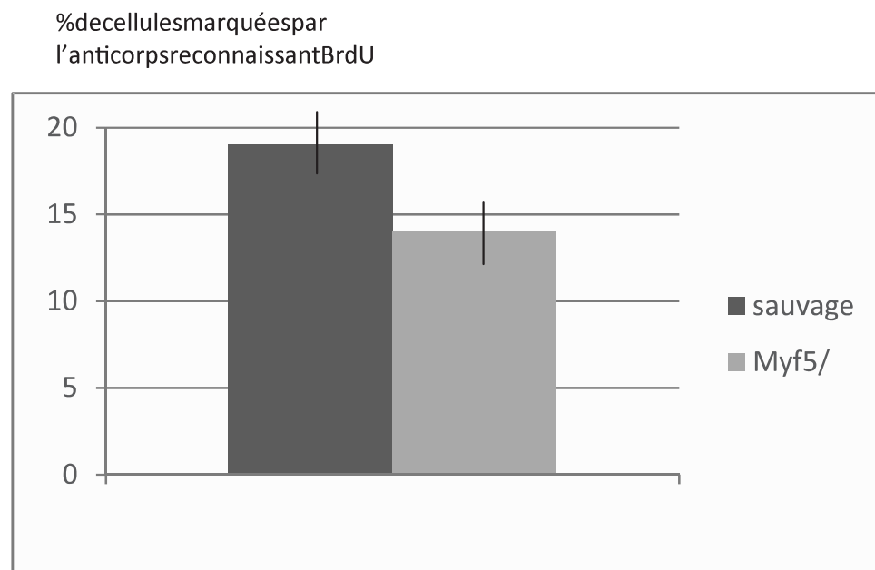
Figure 4 : On détermine le pourcentage de cellules reconnues par l'anticorps anti-BrdU après quelques jours de culture in vitro de fibres musculaires dissociées de MAT de souris sauvages ou mutantes Myf5 -/- âgées de 6 semaines dans un milieu favorisant la prolifération des cellules satellites. Les traits verticaux représentent l'écart-type.
