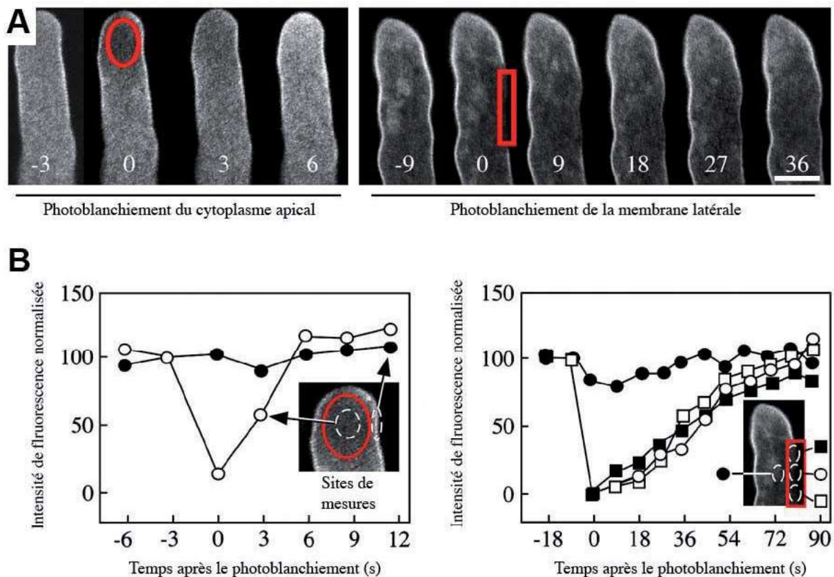
Figure 3 : A. Analyse avec la méthode de photoblanchiment de tubes polliniques exprimant la protéine GFP:PLC1. Les nombres représentent le temps (en seconde) après le photoblanchiment, qui a été effectué dans les zones indiquées en rouge. La série d'images montrée est représentative de 9 expériences indépendantes. La barre indique l'échelle de la photographie et représente 10 \mu\text{m} . B. Analyse quantitative de la récupération après le photoblanchiment. L'intensité de fluorescence a été mesurée dans les régions indiquées (lignes pointillées dans les photographies insérées) avant et après le photoblanchiment des régions définies par les cadres rouges. Les intensités ont été normalisées par rapport à la mesure effectuée juste avant le photoblanchiment.
