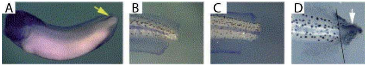
Figure 2 : Hybridations in situ du gène Msx1 . Les flèches indiquent les zones du marquage spécifique de Msx1 . A. Vue latérale de l'embryon au stade 30 orienté avec l'extrémité antérieure à gauche. B. Queue de têtard amputée à 50% au stade 46 et fixée 3 jours plus tard. C. Queue de têtard amputée à 50% au stade 48 et fixée immédiatement. D. Queue de têtard amputée à 50% au stade 48 et fixée 3 jours plus tard. Le niveau d'amputation est indiqué par la ligne noire. La sonde utilisée pour effectuer l'hybridation sur ces 4 photographies est révélée avec un substrat enzymatique faisant apparaître un produit bleu foncé.
