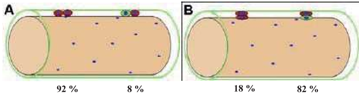
Figure 7 : Schémas résumant les résultats des immunofluorescences Pax7 et YFP sur des fibres musculaires en régénération. On ne représente les résultats que pour des cellules Pax7+ côte à côte, qui sont les deux cellules filles d'une même mitose. Les cellules en rouge n'expriment pas YFP, les cellules vertes expriment YFP. On classe en A ou en B, les cellules filles d'après leur position relative par rapport à la membrane basale (ligne verte) et la fibre musculaire (beige). Dans chacune de ces catégories (A ou B) on montre les proportions des couples où les deux cellules n'expriment pas YFP et où l'une des cellules expriment YFP. On ne tient pas compte dans ces statistiques des cas où les deux cellules expriment YFP.
