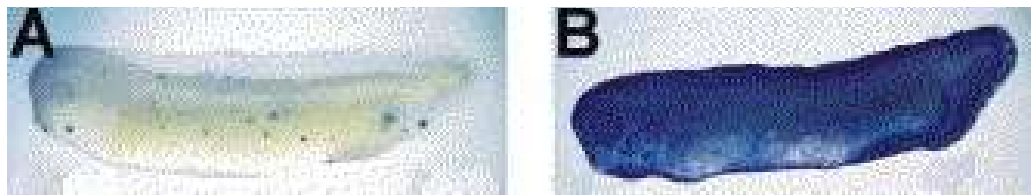
Figure 3 : Embryons transgéniques exprimant une protéine étiquetée Myc sous le contrôle du promoteur du gène HSP70 , et ayant subi (B) ou non (A) un traitement à 34°C pendant 30 minutes au stade 14. L'expression du transgène est visualisée par immunomarquage à l'aide d'un anticorps spécifique dont la présence est révélée à l'aide d'une réaction enzymatique faisant apparaître un produit bleu foncé sur les photographies.
