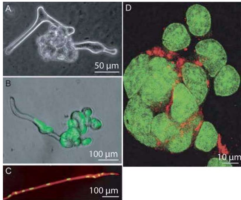
Figure 6 : A. Photographie d'une myofibre 48 heures après son adhérence à la surface de la boîte de culture. B. Photographie prise au microscope d'une myofibre 72 heures après son adhésion. La cellule a été marquée avec un marqueur fluorescent vert qui colore le noyau. C. Photographie prise au microscope à fluorescence 24 h après la microinjection du « TR-dextran ». La cellule a été marquée avec le marqueur fluorescent vert qui colore les noyaux. D. Photographie prise au microscope à fluorescence d'une colonie formée à partir d'une seule myofibre injectée 48 h plus tôt avec le marqueur « TR-dextran ». Les cellules ont été marquées avec le marqueur fluorescent vert qui colore les noyaux.
