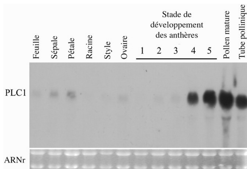
Figure 1 : Analyse par Northern blot du gène PLC1 . Vingt microgrammes d'ARN total de Petunia ont été isolé de chaque tissu indiqué en haut de la photographie ainsi qu'à partir de grains de pollen et de tubes polliniques. Ces ARN ont ensuite été chargés dans chaque puits. Les ARN ont ensuite été transféré sur une membrane en nylon et une sonde radiomarquée provenant de l'ADNc PLC1 a été utilisée pour la révélation. La coloration au bromure d'éthidium du gel (tâches claires) montre les bandes qui correspondent aux ARN ribosomiaux (ARNr). Différents stades de développement des anthères ont également été utilisés : développement des microspores dans la configuration en tétrade (1), microspores uninuclées libres (2), microspores binuclées (3), microspores trinucées (4) et pollen mature (5).
