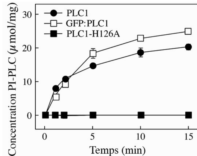
Figure 4 : Dosages biochimiques pour déterminer l'activité d'hydrolyse du PIP2 des protéines PLC1, GFP:PLC1 et PLC1-H126A. Les résultats représentent la moyenne de 3 expériences et les barres d'erreurs l'écart-type des mesures.
