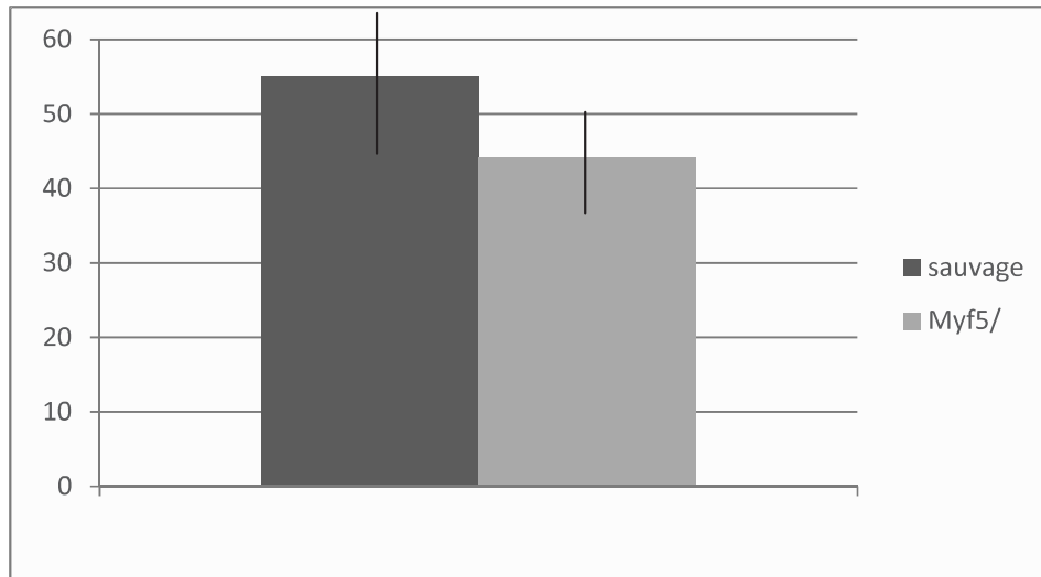
Figure 3 : On détermine par immunofluorescence le nombre moyen de cellules exprimant Pax7 par coupe de MAT de souris sauvages ou mutantes Myf5 -/- âgées de 6 semaines. Les traits verticaux représentent l'écart-type.
