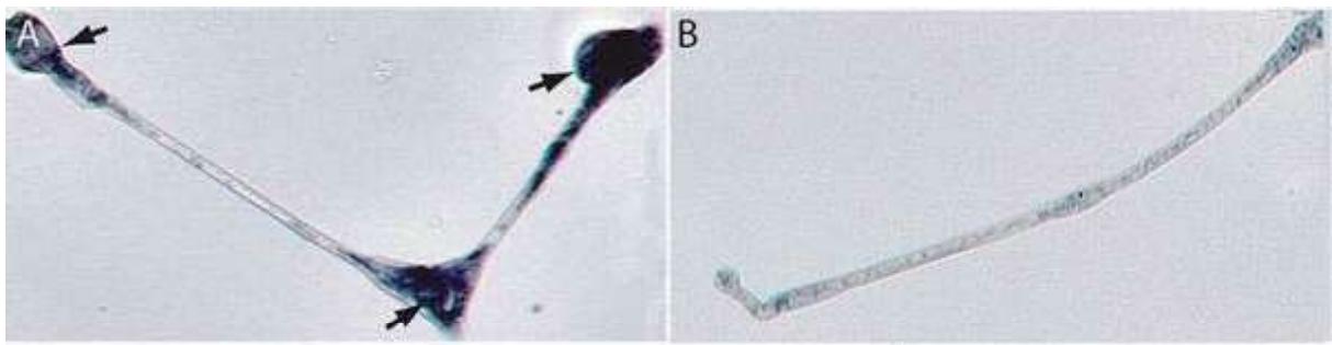
Figure 7 : Photographie après 48 h de cultures de myofibres dissociées. L'expression de l'ARNm du gène Msx1 est détecté par hybridation in situ . La sonde utilisée pour effectuer l'hybridation est révélée avec un substrat enzymatique faisant apparaître un produit bleu foncé. A. Vue d'une myofibre qui montre des parties en forme d'amas globulaire (flèches). B. Photographie d'une myofibre qui conserve un aspect normal. Les deux images proviennent de la même culture.
