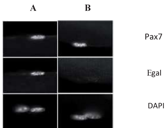
Figure 5 : Immunofluorescences réalisées sur des coupes de MAT de souris hétérozygotes Myf5 LacZ / Myf5 + âgées de 6 semaines. Sur une colonne (A ou B) on observe les mêmes cellules avec des marquages différents (Pax7 sur la première ligne, E-galactosidase sur la deuxième ligne et DAPI (qui marque l'ADN) sur la dernière ligne). Les colonnes A et B présentent les résultats pour
