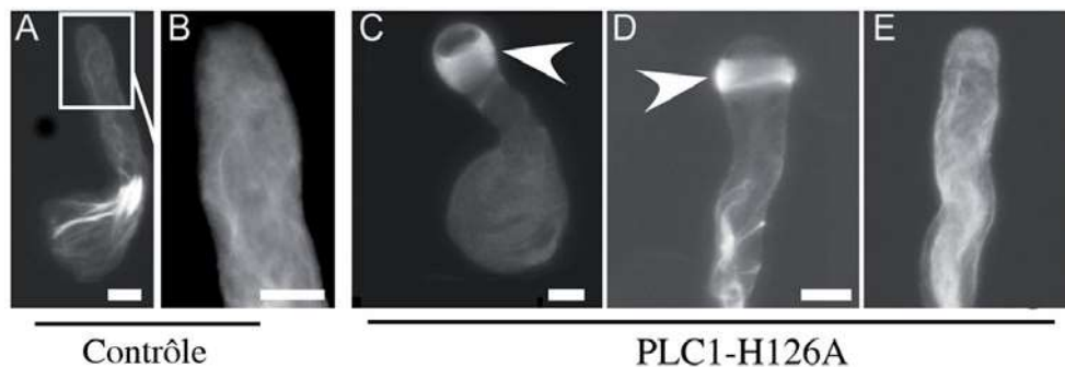
Figure 5 : La distribution de l'actine est suivie à l'aide de la protéine GFP:mTalin dans des tubes polliniques contrôles (A, B) et dans des tubes polliniques qui expriment la construction PLC1-H126A de façon transitoire (C, D). La flèche blanche pointe une structure que l'on observe avec PLC1-H126A mais pas chez le contrôle. La dernière figure de droite (E) correspond à la visualisation du réseau d'actine quand les grains de pollens exprimant la PLC1-H126A ainsi que la GFP:mTalin sont mis à germer sur un milieu contenant 5 nM d'une drogue capable de désorganiser l'actine. La barre indique l'échelle de la photographie et représente 10 μm.
