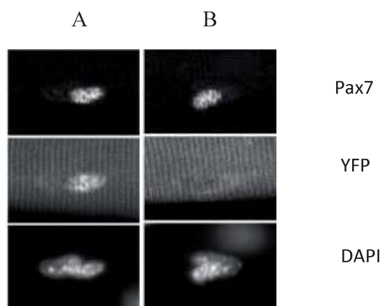
Figure 6 : Immunofluorescences réalisées sur des coupes de MAT de souris Myf5-Cre; ROSA-YFP âgées de 6 semaines. Sur une colonne (A ou B) on observe les mêmes cellules avec des marquages différents (Pax7 sur la première ligne, YFP sur la deuxième ligne et DAPI (qui marque l'ADN) sur la dernière ligne). Les colonnes A et B présentent les résultats pour deux champs d'observation différents sur un même muscle.
