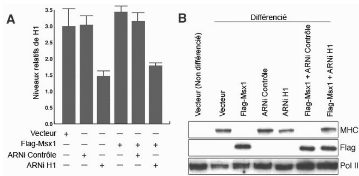
Figure 11. Des cellules C2C12 exprimant la protéine Flag-Msx1 et l'ARN interférent de l'histone H1 (ARNi H1) ou un vecteur contrôle ont été mises en culture dans des conditions permettant ou non la différenciation. A. Quantification de l'ARN codant pour l'histone H1 par PCR. Les histogrammes montrent la moyenne obtenue sur six expériences. Les barres d'erreurs indiquent l'écart-type des mesures. Pour chaque barre sont indiquées en dessous de l'histogramme les différentes constructions exprimées dans les cellules C2C12. B. Résultats obtenus après la migration des protéines par électrophorèse de différents extraits cellulaires de cellules C2C12 exprimant les constructions indiquées en colonnes et révélés par les anticorps indiqués en ligne.
