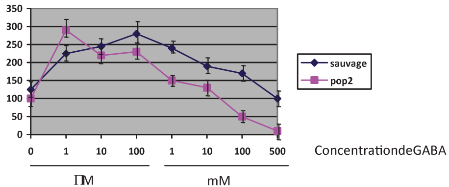
Figure 2 : La longueur des tubes polliniques est mesurée après 16 heures de croissance dans des gels d'agarose dans lesquels on a déposé une concentration donnée de GABA. Les barres verticales représentent les écart-types.
