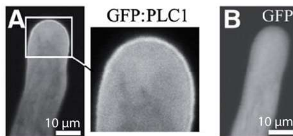
Figure 2 : A et B. Expression de la protéine de fusion GFP:PLC1 (A) ou de la GFP seule (B) dans des grains de pollens après transfection. L'extrémité du tube pollinique est grossie dans la photographie centrale. Les images montrées sont représentatives de plus d'une centaine de tubes polliniques individuels.
