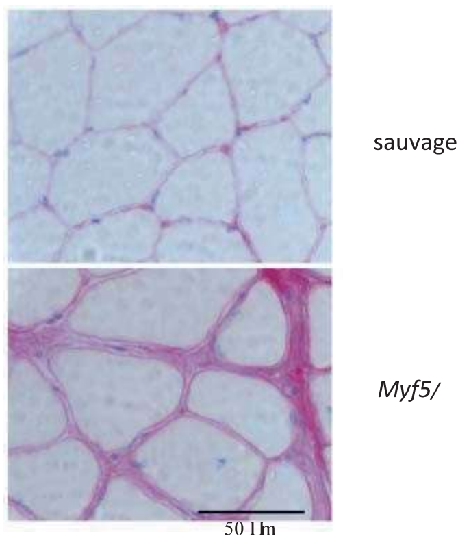
Figure 1 : Coupes transversales de MAT de souris sauvages ou mutantes Myf5 -/- traitées par le rouge Sirius qui colore en rose la matrice extracellulaire (collagène de type I et III) et par le DAPI qui colore en bleu-violet les noyaux cellulaires. L'échelle est la même pour les deux images.
