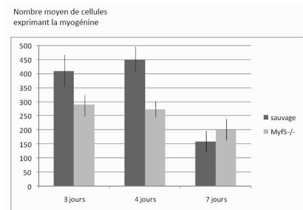
Figure 2 : On détermine par immunofluorescence le nombre moyen de cellules exprimant la myogénine par coupe de MAT dans la région lésée 3, 4 ou 7 jours auparavant par l'application d'un objet métallique à -196°C. Les traits verticaux représentent l'écart-type.
