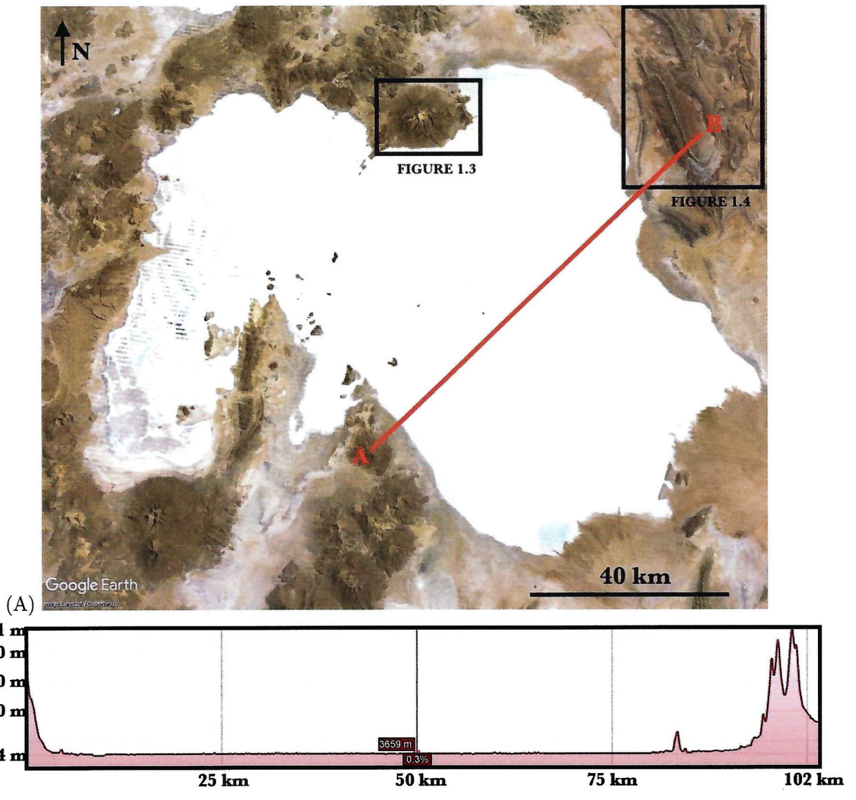
FIGURE 1.2. – (A) Image satellite acquise par la constellation de satellites Landsat du salar d’Uyuni. Le trait rouge localise le profil topographique Sud Ouest – Nord Est. Les cadres localisent les FIGURE 1.3. et FIGURE 1.4. . (B) Profil topographique Sud Ouest – Nord Est du salar d’Uyuni (attention les échelles horizontale et verticale sont différentes). Droits réservés : Google Earth , 2024, modifié.
