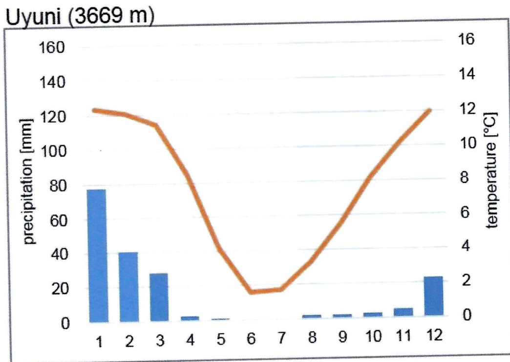
FIGURE 1.6. – Diagramme ombrothermique de la zone d'Uyuni (altitude : 3669 m). Histogrammes bleus = précipitations, courbe orange = températures. Schmidt, 2019.
