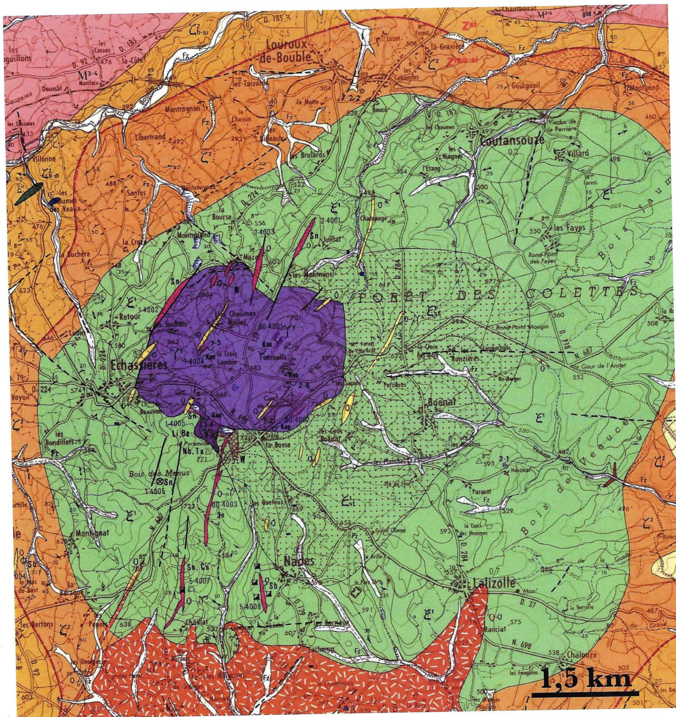
FIGURE 1.1. – Extrait de la carte géologique de Gannat au 1/50 000 ème . Droits réservés : BRGM.
