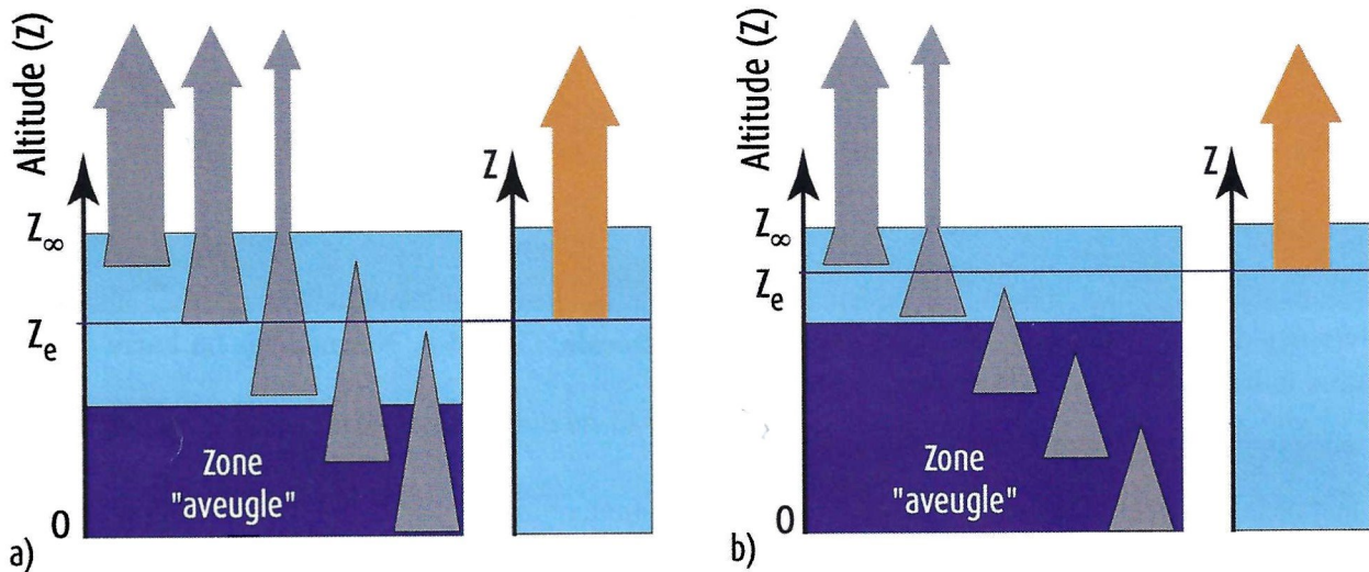
FIGURE 3.3. – Pour les deux figures a) et b), à gauche, représentation schématique de l'évolution du rayonnement émis vers le haut par la surface et par l'atmosphère pour 4 altitudes. La surface est à l'altitude 0 et le sommet de l'atmosphère à l'altitude Z ∞ . Les formes en triangle schématisent la diminution progressive de l'intensité du rayonnement avec l'altitude, du fait de l'absorption par l'atmosphère, pour un rayonnement émis à la base du triangle. À droite, en orange, représentation de l'altitude d'émission correspondante.
