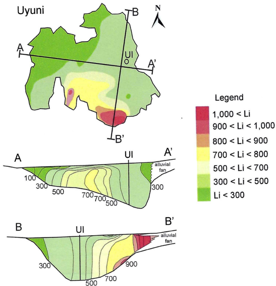
FIGURE 1.5. – Courbes d'isoconcentration en Li des saumures du salar d'Uyuni en \text{mg.L}^{-1} et coupes dans le salar. Steinmetz et Salvi, 2021.
