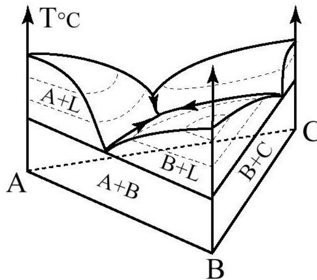
Principe général du diagramme ternaire à eutectique
