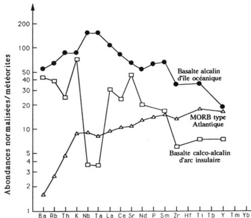
Abondance des éléments-traces pour les tholéiites (MORB), les basaltes alcalins des îles (OIB) et les basaltes calco-alcalins des arcs insulaires (Spiderdiagram)
