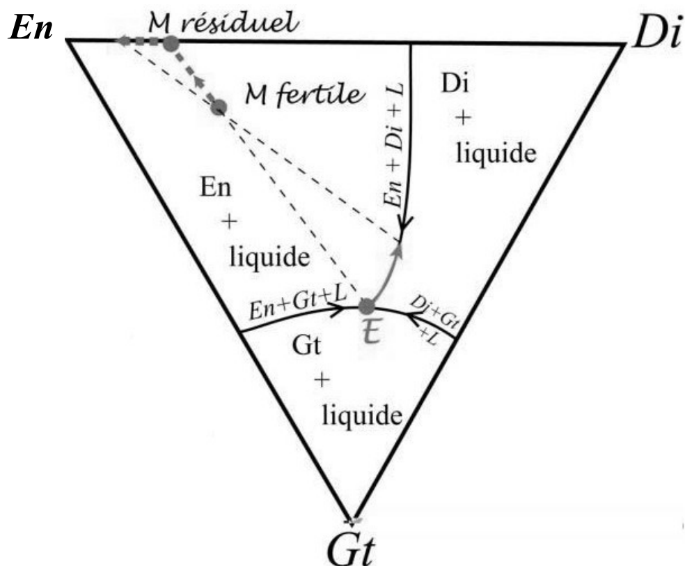
Principe général du diagramme ternaire à eutectique
