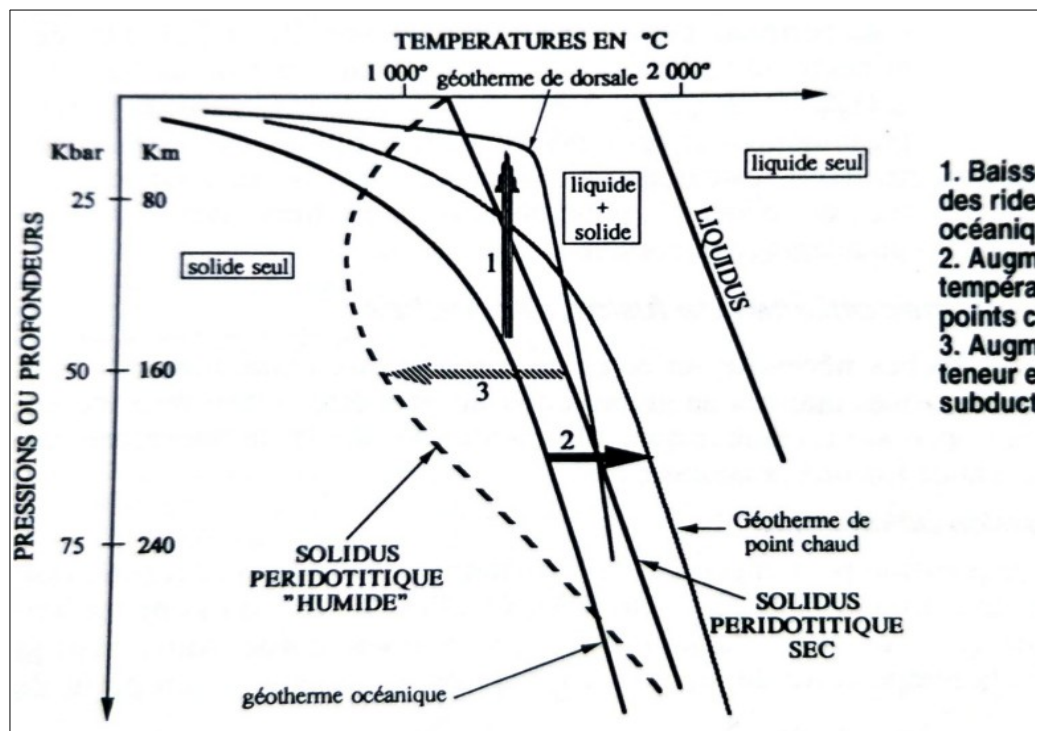
Fusion partielle et contextes géodynamiques
