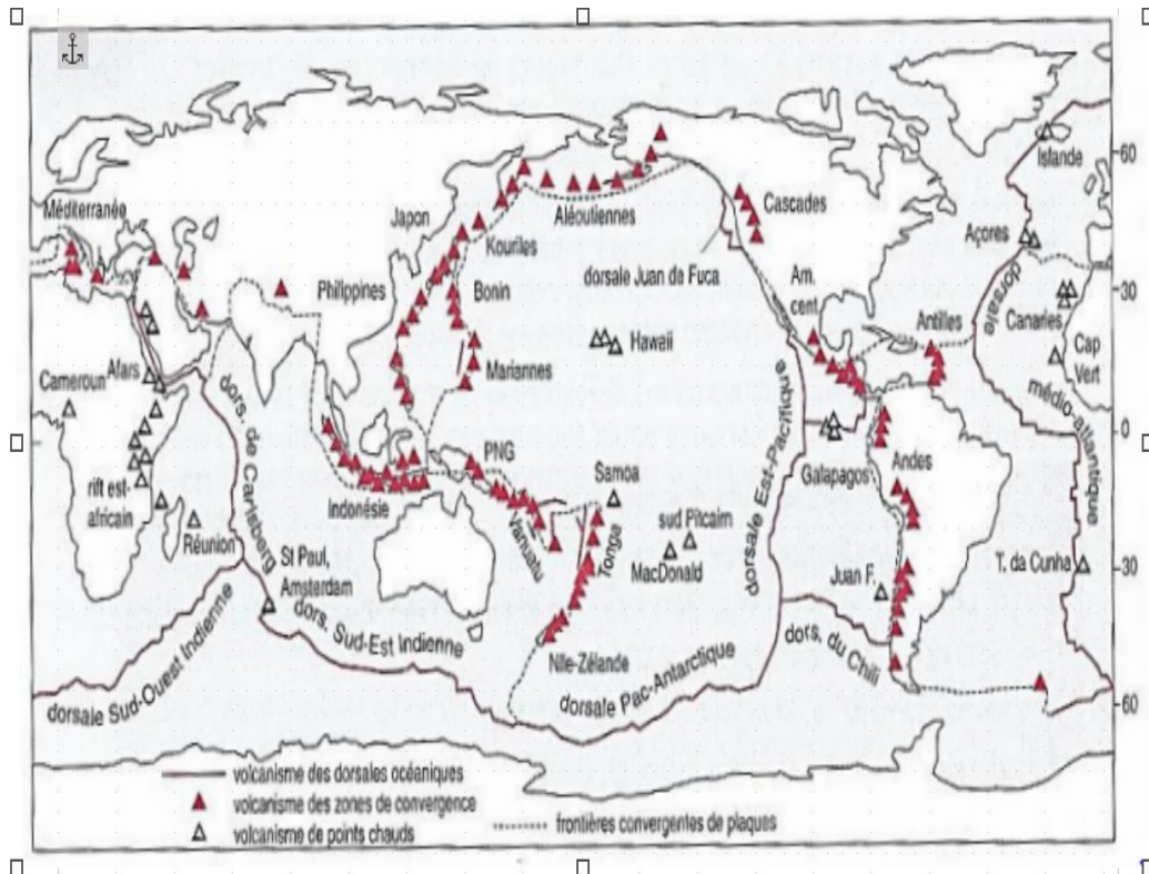
document 2 : différences entre les deux grandes catégories de volcans
