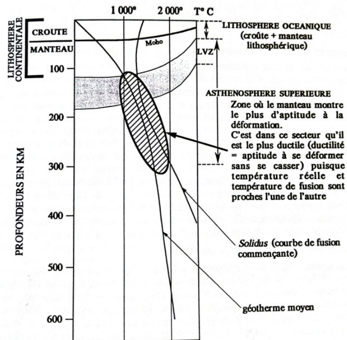
Géotherme, solidus des péridotites et « fenêtre de fusion partielle »
