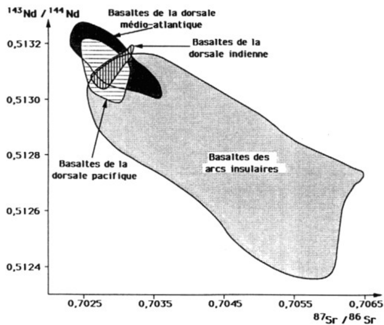
Variations isotopiques de Nd et Sr des basaltes des dorsales comparées à celles des basaltes des arcs insulaires
