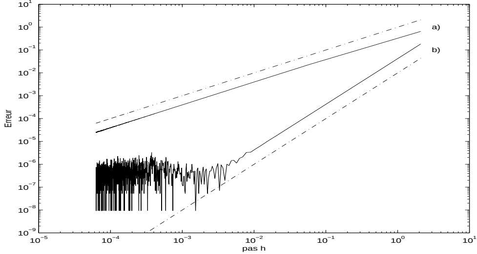
Figure 1: Erreur entre l'intégrale I et son approximation par une formule de quadrature pour la fonction f(x) = x^4 sur l'intervalle [0, 2\pi] , en fonction du pas h . Le pas local h_i est constant et égal à h = \frac{2\pi}{N} . Les deux axes sont en échelle logarithmique. a): en trait plein l'erreur mesurée pour la formule des rectangles et en pointillé la courbe y = h . b): en trait plein l'erreur mesurée pour la formule des trapèzes et en pointillé la courbe y = h^2/100 .
