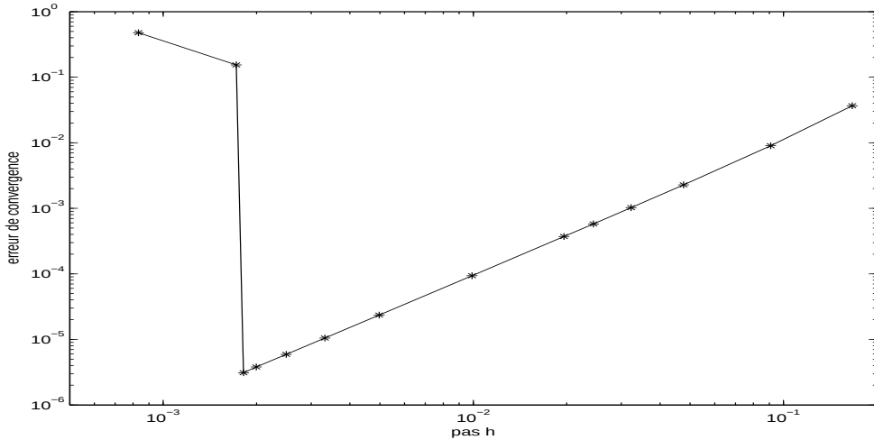
Figure 2: Erreur en norme Euclidienne entre la solution exacte U et son approximation \mathcal{U}_N par la méthode de différences finies, en fonction du pas h = 1/N . Les deux axes sont en échelle logarithmique. On a résolu l'équation (37) avec f(x) = -2\pi \sin(\pi x) + \pi^2(1-x)\cos(\pi x) ce qui donne comme solution exacte U(x) = (1-x)\cos(\pi x) .
