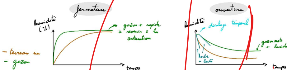
Figure 8 – Tendances schématisées des variations d'humidité
