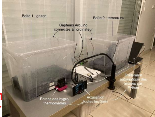
Figure 6 – Montage de la 1 re expérience (le gazon n'a pas encore poussé)
