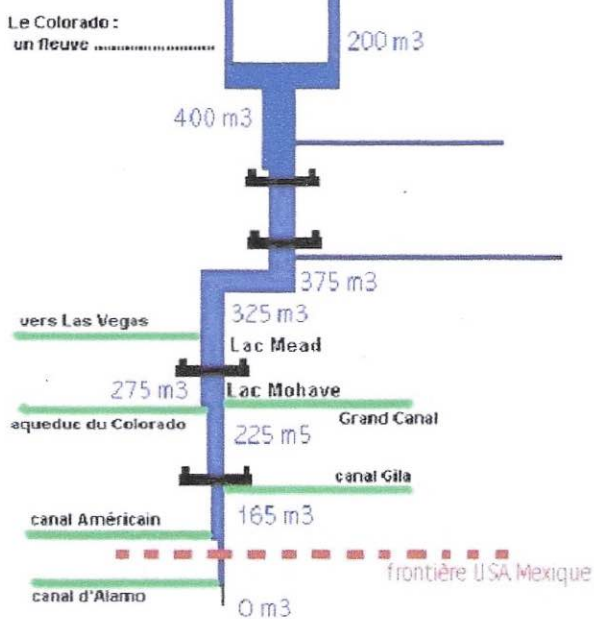
Schéma des barrages sur le Colorado et débits
