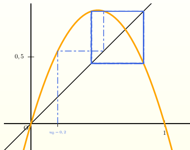
Figure : u_{n+1} = 3, 4u_n(1 - u_n) avec u_0 = 0, 2 .
