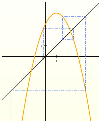
Figure : u_{n+1} = (u_n + 1)(3 - u_n) avec u_0 = -0.2 . f a deux points fixes et (u_n)_{n \in \mathbb{N}} diverge vers -\infty .
