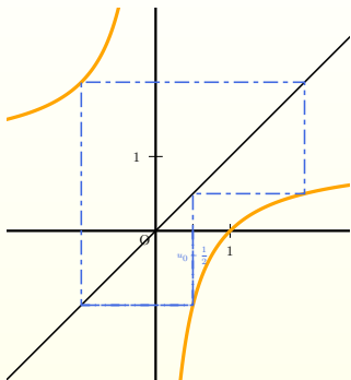
Figure : u_{n+1} = 1 - \frac{1}{u_n} avec u_0 = \frac{1}{2} .
