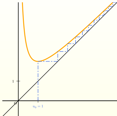
Figure : u_{n+1} = u_n + \frac{1}{u_n} avec u_0 = 1 . f n'a pas de points fixes et (u_n)_{n \in \mathbb{N}} diverge vers +\infty .
