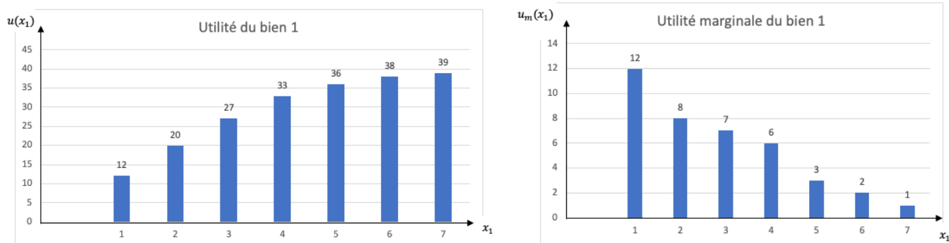
Figure 1 : Utilité totale et Utilité marginale du bien 1
