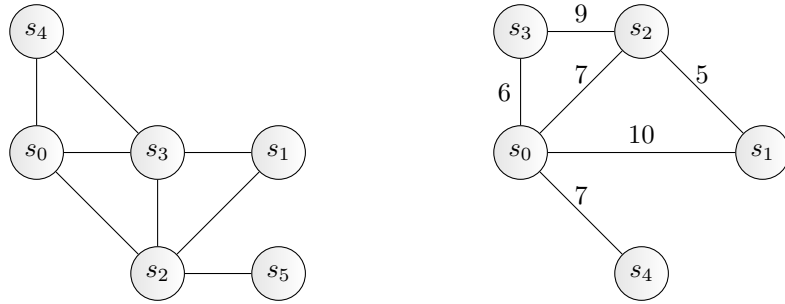
FIG. 3 – Les graphes G_1 et G_2
