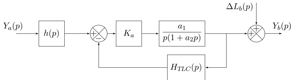
FIGURE 4 – Modèle de commande en mode « Recentrage »
