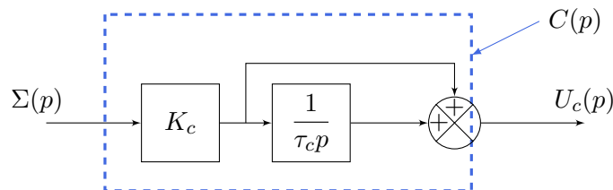
FIGURE 6 – Schéma-blocs du correcteur C(p)
