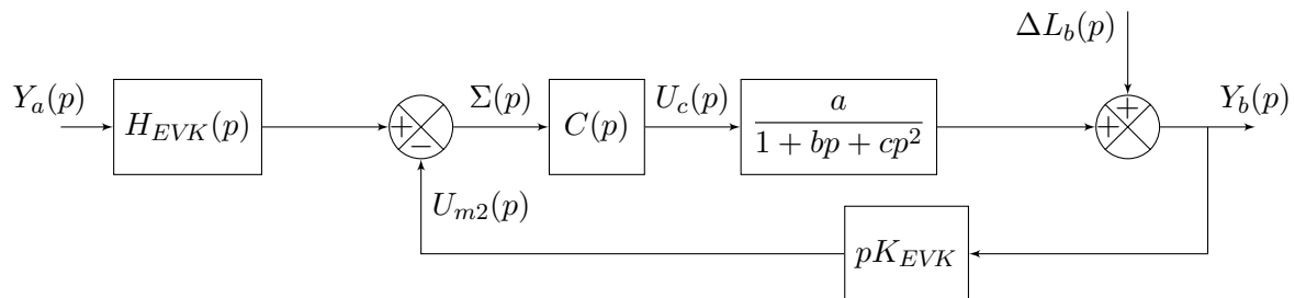
FIGURE 5 – Modèle de commande en mode « Automatique »
