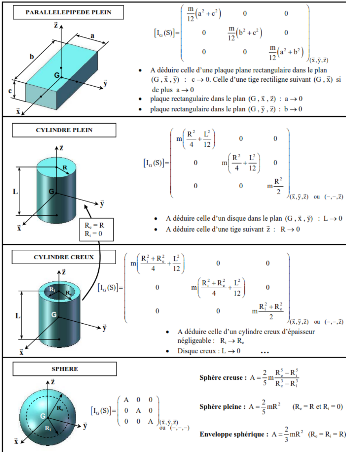
FIGURE 2 – Matrice d'inertie des solides usuels au centre d'inertie G
