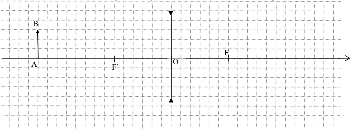
Lentilles minces - construction de l'image d'un objet
