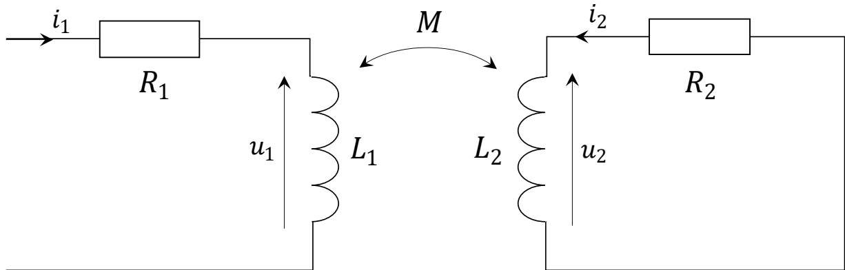
Figure 8 - Circuit équivalent au système solénoïde central – plasma
