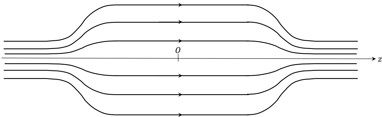
Figure 3 - Lignes de champ d'une bouteille magnétique
