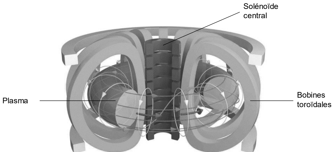
Figure 2 - Schéma d'un tokamak
