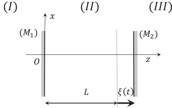
FIGURE 2 – Cavité résonante à miroir mobile (partie 2).
