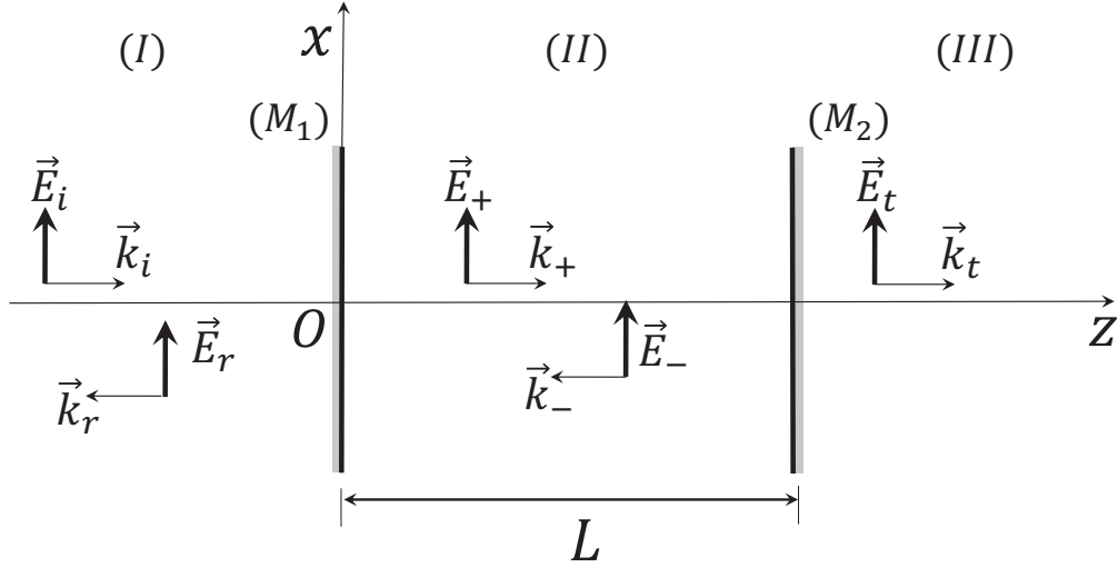
FIGURE 1 – Cavité résonante linéaire de longueur L , soumise à un champ incident (partie 1).
