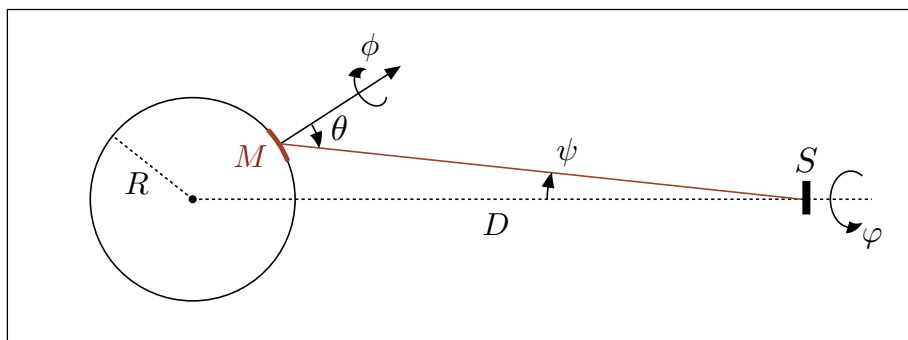
FIGURE 2 – Détection du rayonnement d'un corps céleste.
