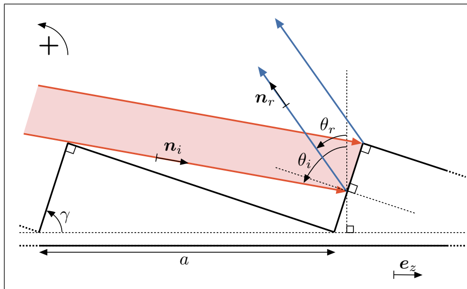
FIGURE 7 – Schéma d'un motif de réseau en réflexion blazé.
