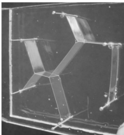
FIG. 2 – Films de savon reliant des tiges métalliques entre deux plaques de plexiglas. Il y a trois sommets intermédiaires. 2
