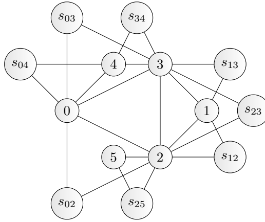
FIG. 6 – Une représentation de G'_1 . Pour simplifier, on a renommé chaque sommet s_i par i .
