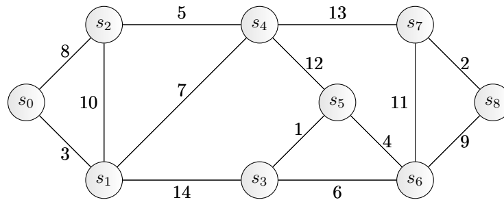
FIG. 4 – le graphe pondéré G_3
