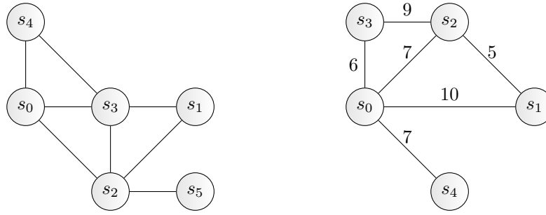
FIG. 3 – Les graphes G_1 et G_2
