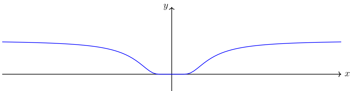
FIGURE 3 – Graphe de f , fonction plate en 0
