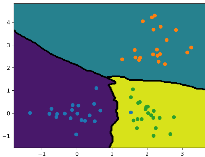
FIGURE 2 – Zones délimitées par les k plus proches voisins
