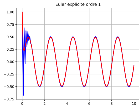
FIGURE 2 – Méthode d'Euler explicite
