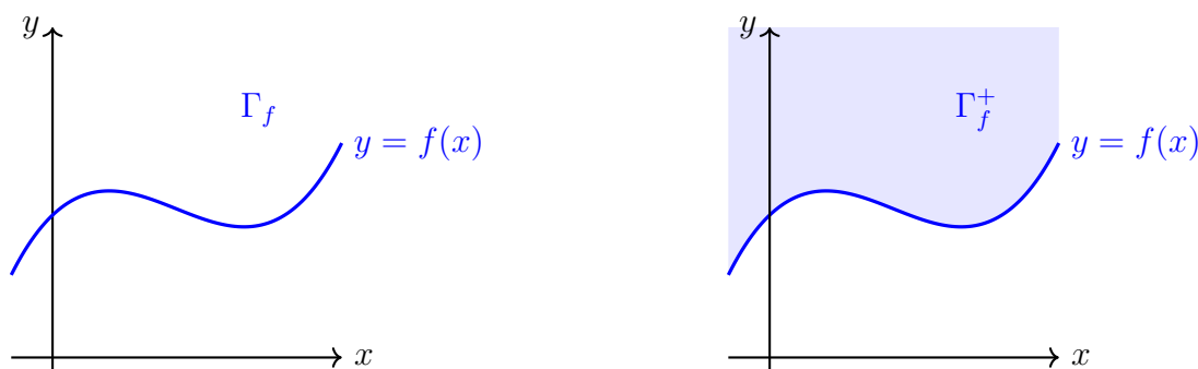
FIGURE 3 – Graphe et épigraphe de f
