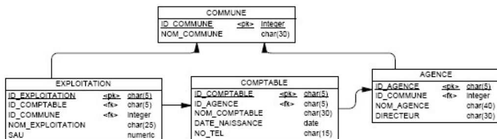
Modèle logique des données
