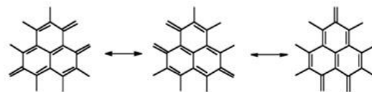
(3) Mésomérie au sein d'un feuillet
