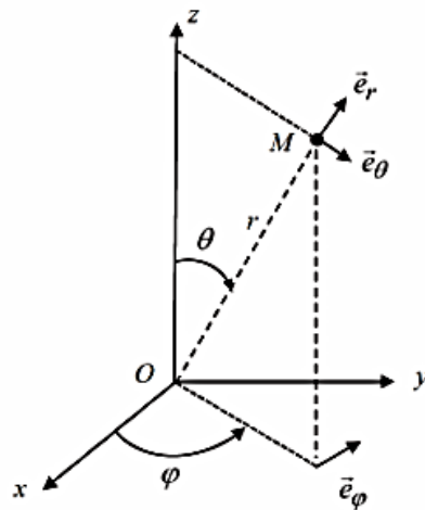
Figure 3 - Coordonnées sphériques
