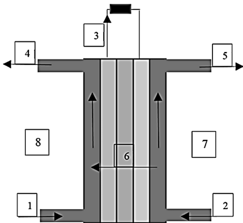
Figure 3 - Schéma de la pile à combustible SOFC
