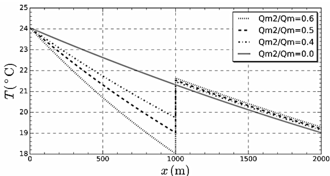
Figure 14 Champ de température au sein des logements
