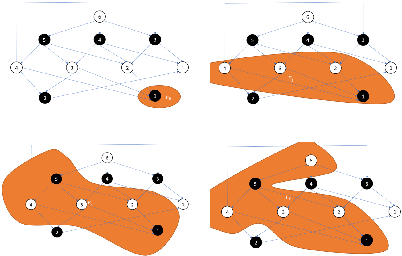
CALCUL DE L'ATTRACTEUR DU COUPLE (F_0, J_0) QUI EST F_3
