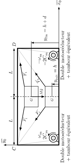
Figure 5 Modèle d'étude du déplacement vertical de la plate-forme en position centrée dans le plan médian sous l'action des deux câbles équivalents supérieurs (l'influence des deux câbles équivalents inférieurs est négligée et ils ne sont donc pas représentés)
