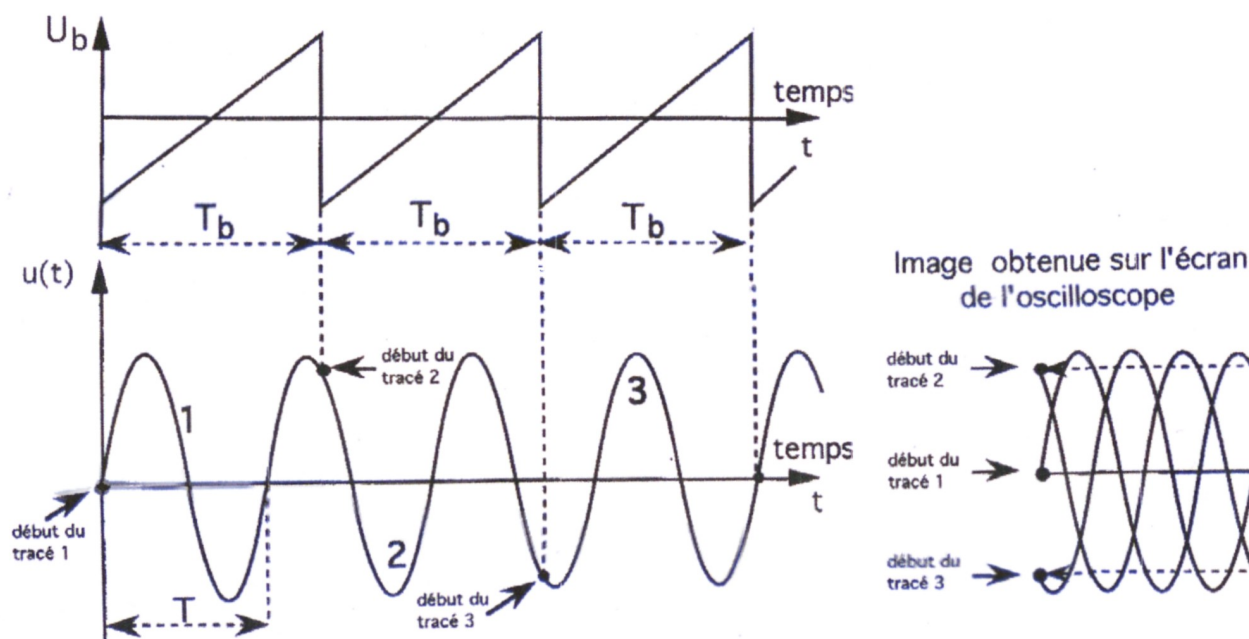
Figure 1 : u_b = base des temps = tension en dents de scie T_b = temps de balayage de l'écran u(t) : tension à mesurer.
