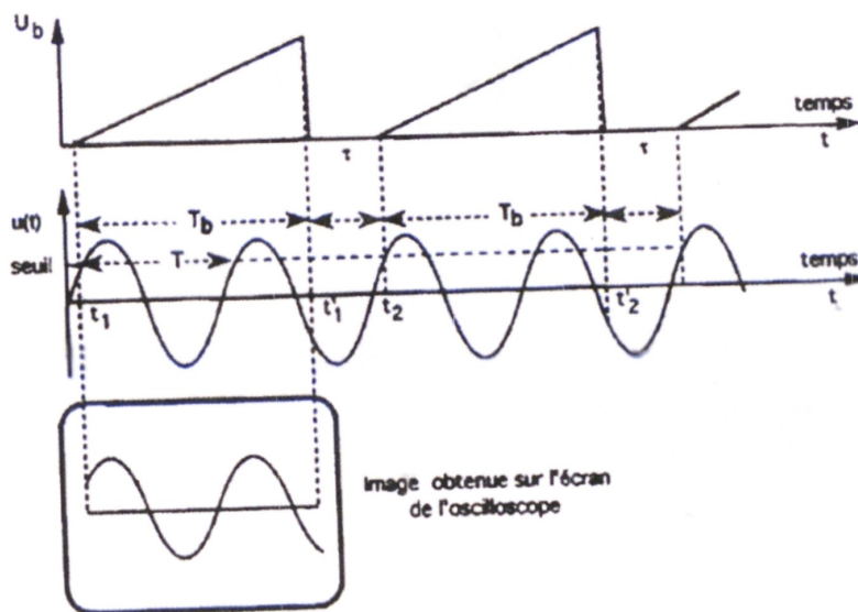
Figure 2: Le spot suit alors le même parcours que les courbes précédemment affichées. On peut aussi choisir sur l'oscilloscope la valeur de la d.d.p qui démarre le balayage: elle est appelée valeur du seuil de déclenchement .
