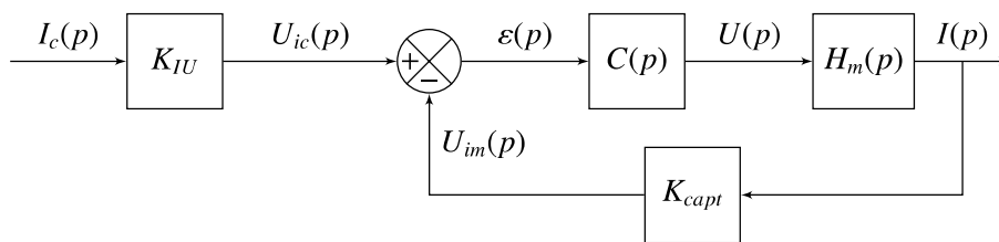
Figure 13 - Schéma bloc de l'asservissement en intensité
