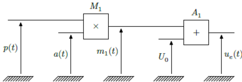
Figure 9 Schéma du circuit de réalisation de u_e(t)
