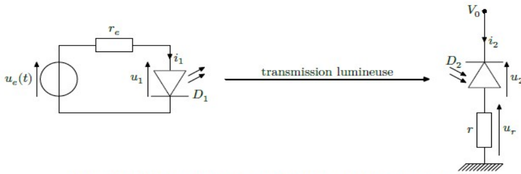
Figure 8 Principe de la transmission d'information par la lumière.
