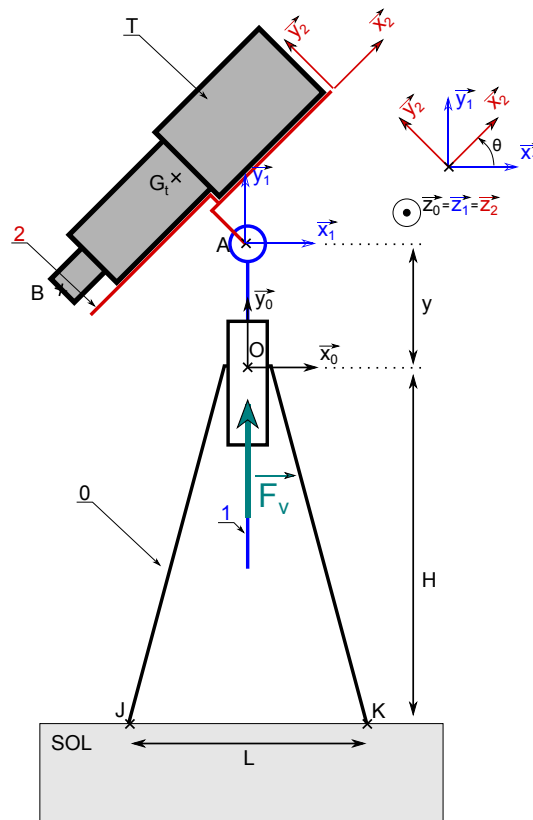
Figure 2: Modèle de prédimensionnement pour le trépied motorisé
