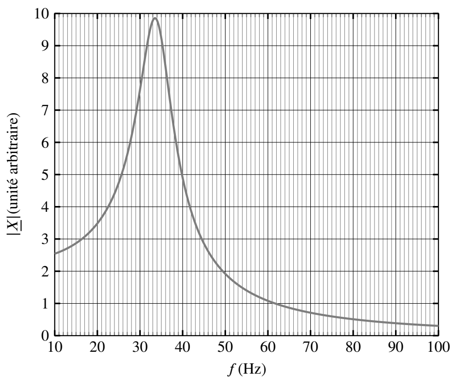
Figure C – Évolution de |X| en fonction de la fréquence d'excitation f .
