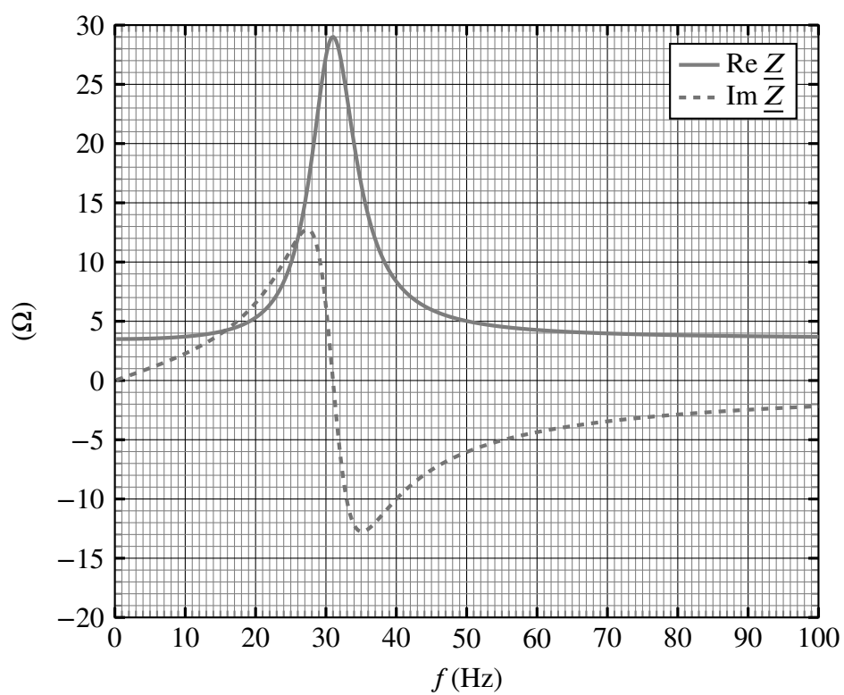
Figure B – Évolution des parties réelles et imaginaires de \underline{Z} en fonction de la fréquence d'excitation f .
