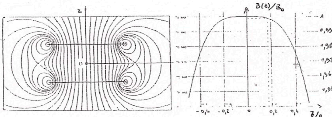
BOBINES DE HELMHOLTZ
