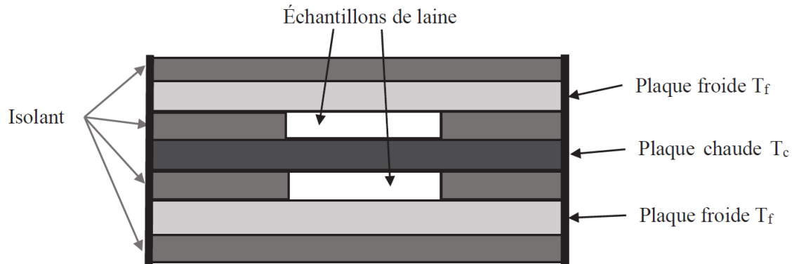
Figure 2 - Principe de la plaque chaude gardée
