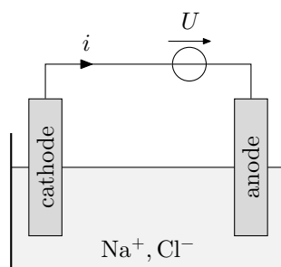
Figure 3: Électrolyseur
