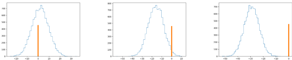
Figure 1.4 – Le trait plein représente la valeur attendue. De gauche à droite : z = 0,5 , z = 2 et z = 5 . Si le z-score devient trop grand (à droite), les valeurs ne sont plus compatibles.
