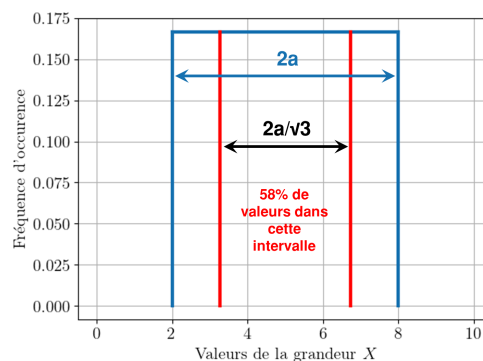
Figure 1.2 – Distribution des valeurs possibles de la grandeur X selon une loi de probabilité uniforme.
