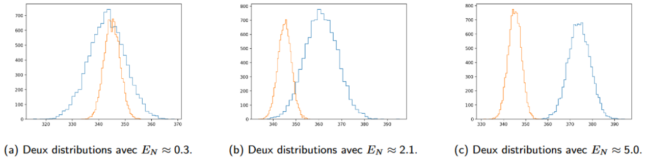
Figure 1.3 – Tracés de trois jeux deux distributions de résultats de mesure avec différents z-score ( E_N ).
