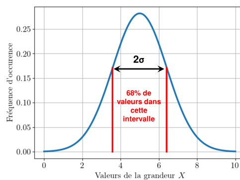
Figure 1.1 – Distribution des valeurs possibles de la grandeur X selon une loi de probabilité gaussienne.
