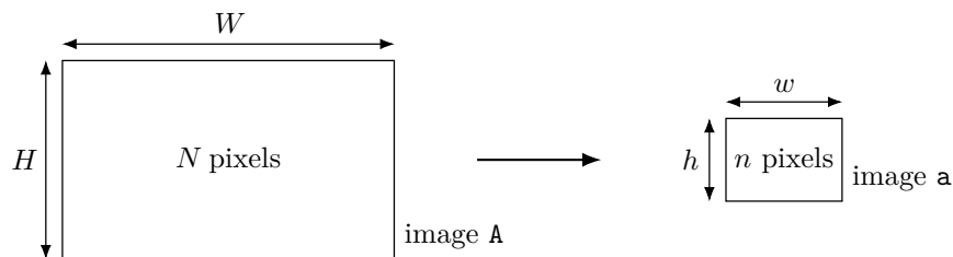
Figure 3 Redimensionnement d'image
