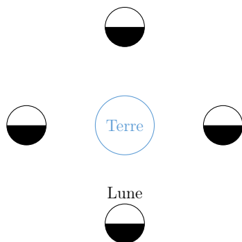
Translation circulaire Pas de face cachée
