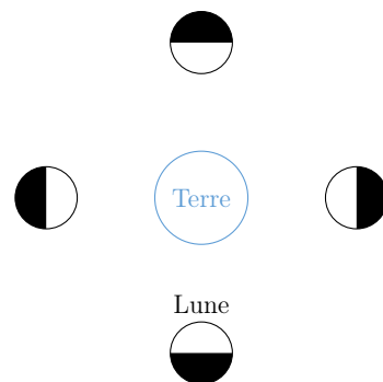
Rotation La Lune a une face cachée
