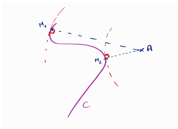
FIGURE XV.4 – Distances extrêmes d'un point à une courbe
