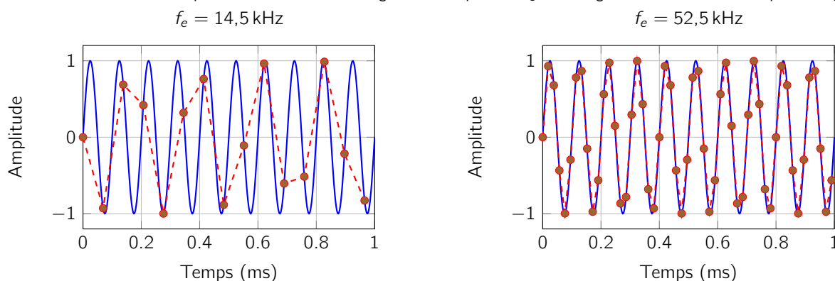
Figure 1 – Différents échantillonnages d'un même signal sinusoïdal. Le signal a pour fréquence f_0 = 10,0 kHz. Les fréquences d'échantillonnage correspondant aux deux figures valent respectivement 14,5 kHz et 52,5 kHz.
